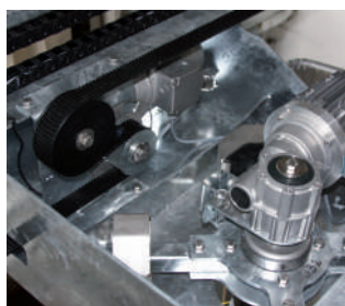
Cinghia di traslazione diretta
