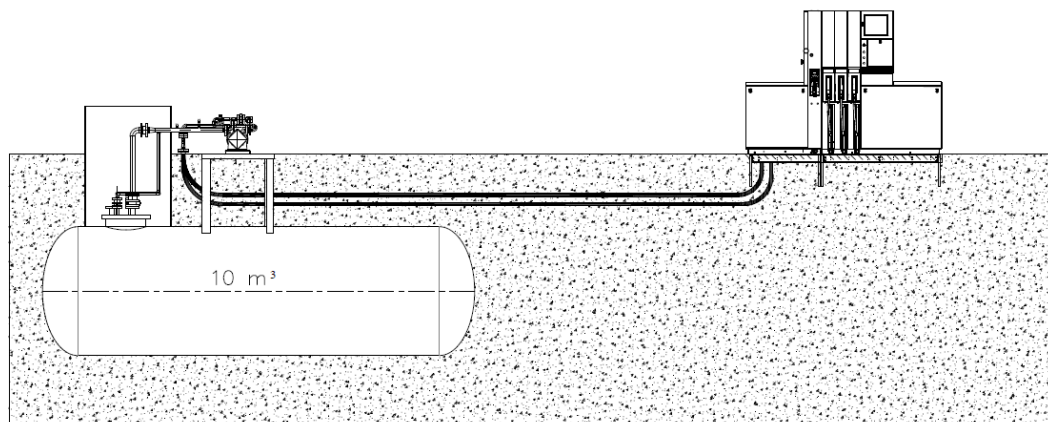
Tip A: Instalacija s podzemnim spremnikom 10m 3
